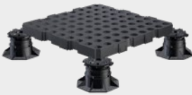
SYSTEM TRIAS WABIC 2.0 Unterkonstruktion für Terrassen
