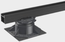
SYSTEM TRIAS ALU Unterkonstruktion für Terrassen
